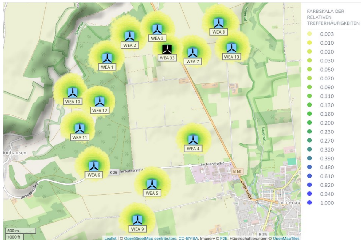
Abbildung A.1.1: Trefferhäufigkeiten von Eisstücken pro Rasterfläche (16m 2 ) und Jahr in der Umgebung der WEA 1 - 13 und der WEA 33 am Standort Lichtenau (Karte /1.4/).
