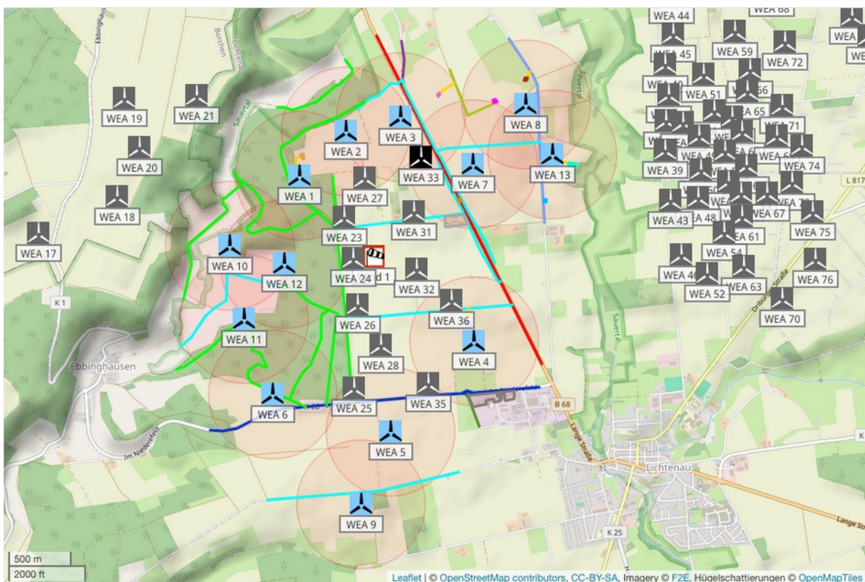
Abbildung 4.3.1: Potentielle Gefährdungsbereiche der WEA und Schutzobjekte am Standort Lichtenau (Karte /1.4/).
